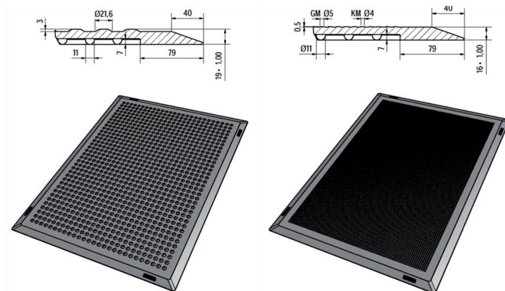
Kupolás felszínű szőnyeg nedves munkaterületre
